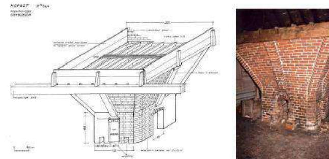
Figuur 5: Oven, hel en eestvloer van hopast De Schepper in Erembodegem (tekening en foto R. De Meerleer, Burst). bron Bécuwe F. & Vandermarlière G.: p. 155, p. 153
