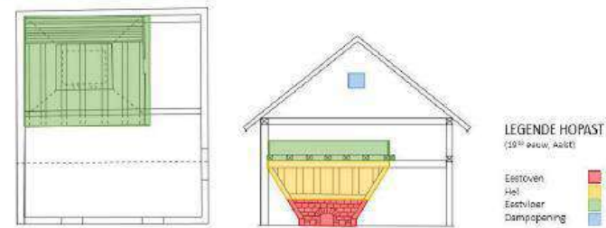
Figuur 4: Bewerkt grondplan en snede van hopast uit de streek van Aalst, zoals beschreven door Samuel von Crauner in 1820 bron Bécuwe F. & Vandermarlière G.: p. 152
